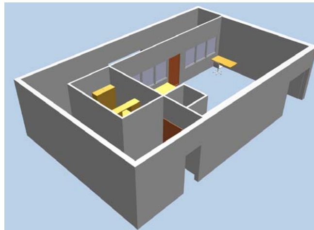
Bild: Layout Reinraum
